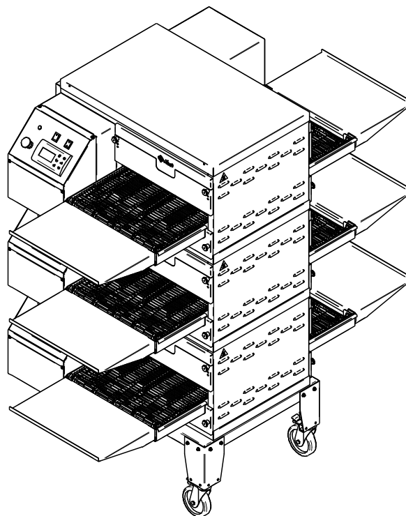
Рис.4 Вариант установки печи ПЭК-400 в три яруса на подставку ПП-400-01
