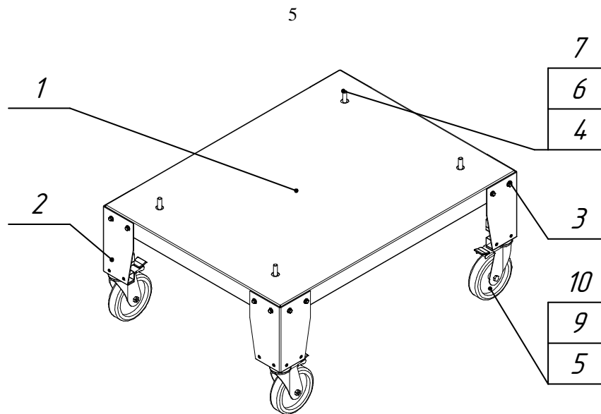
Рис. 6. Схема сборки ПП-400-01
