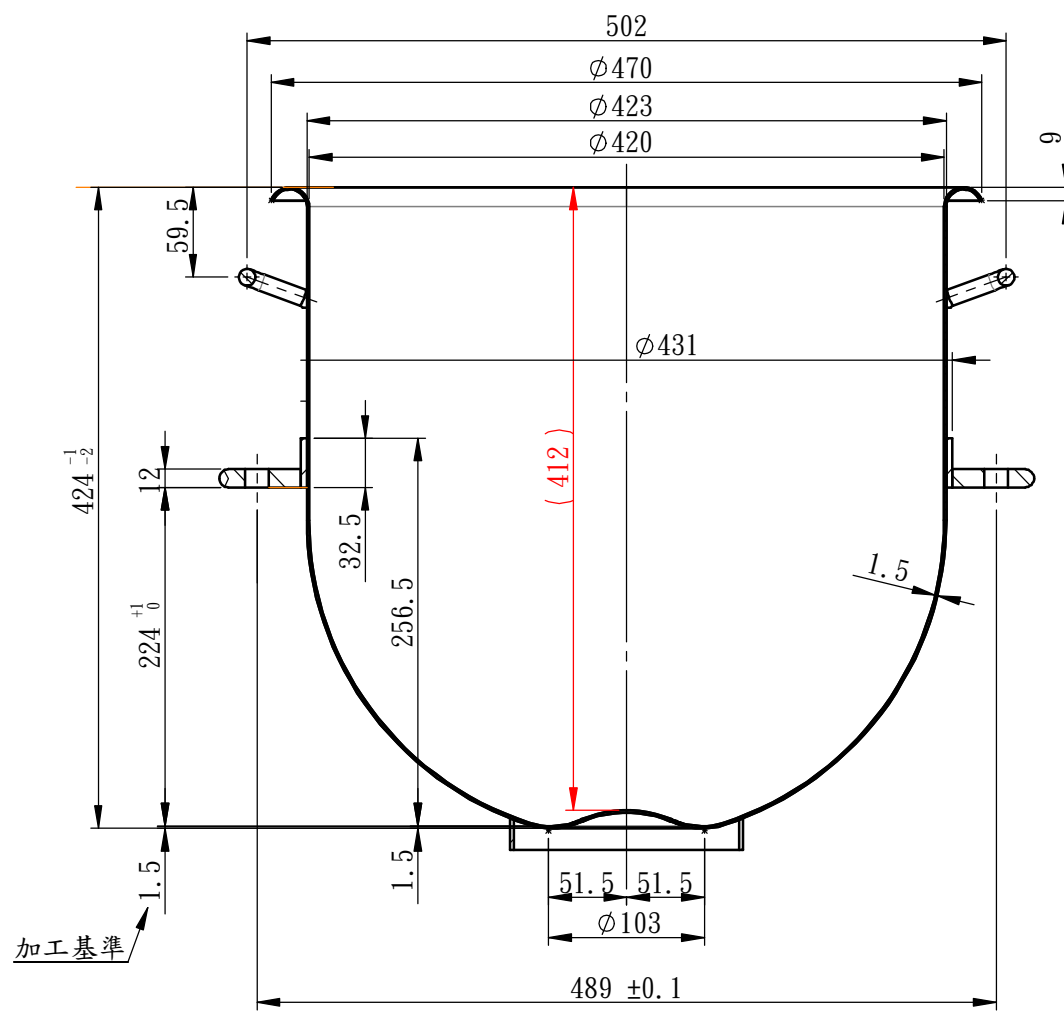
剖面圖 A-A
